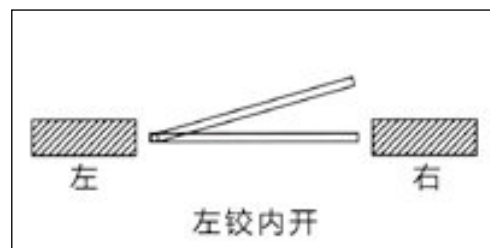
平开门（内开）的锁向图示
